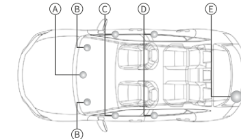
(A) 9cmスコーカー (B) コアキャナル 9cmスコーカー + 2.5cmツイーター (C) 8×9inchウーハー (D) 16cmダブスピーカー (E) 20cmサブウーハー
