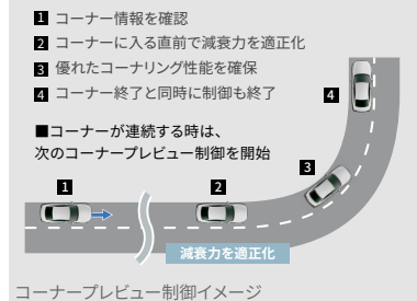
コーナープレビュー制御イメージ
