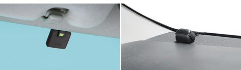
ETCアンテナ装着例 光ビーコンユニット装着例
